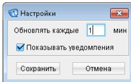
Рис. 15. Окно "Настройки"
